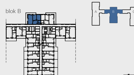
s c h é m a p ů d o r y s u 4 . N P / s c h e m e o f t h e f o u r t h f l o o r
